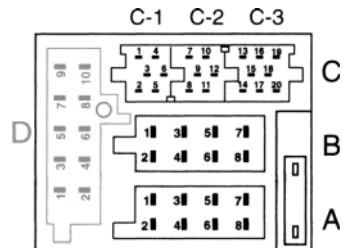
ISO-Anschlüsse des Radios
